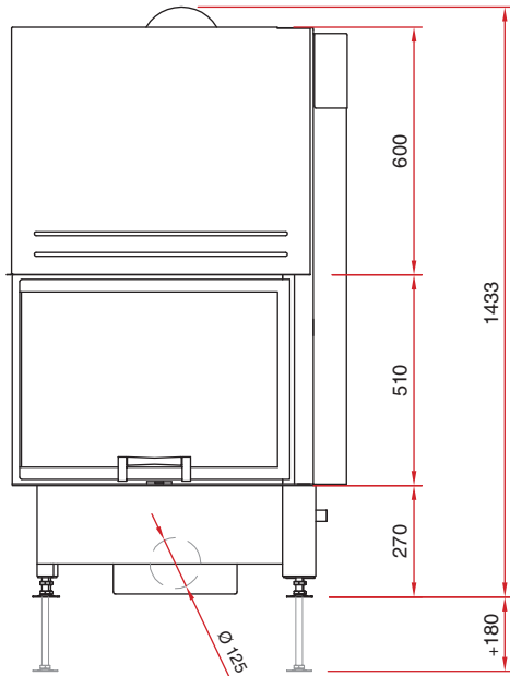
Frontansicht M 1:20
