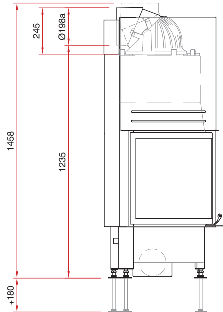
Seitenansicht M 1:20
