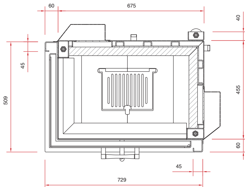
Grundriss M 1:10
