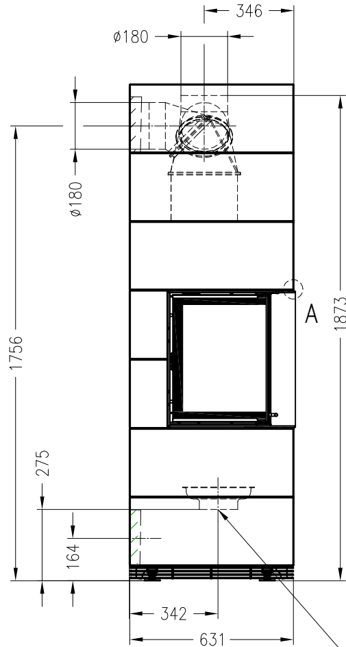
Seitenansicht M~1:20
