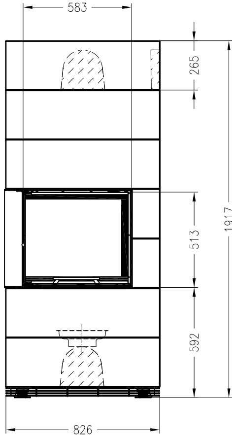
Vorderansicht M~1:20
