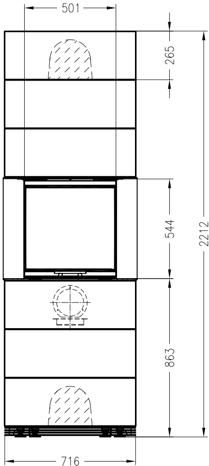
Vorderansicht M~1:20
